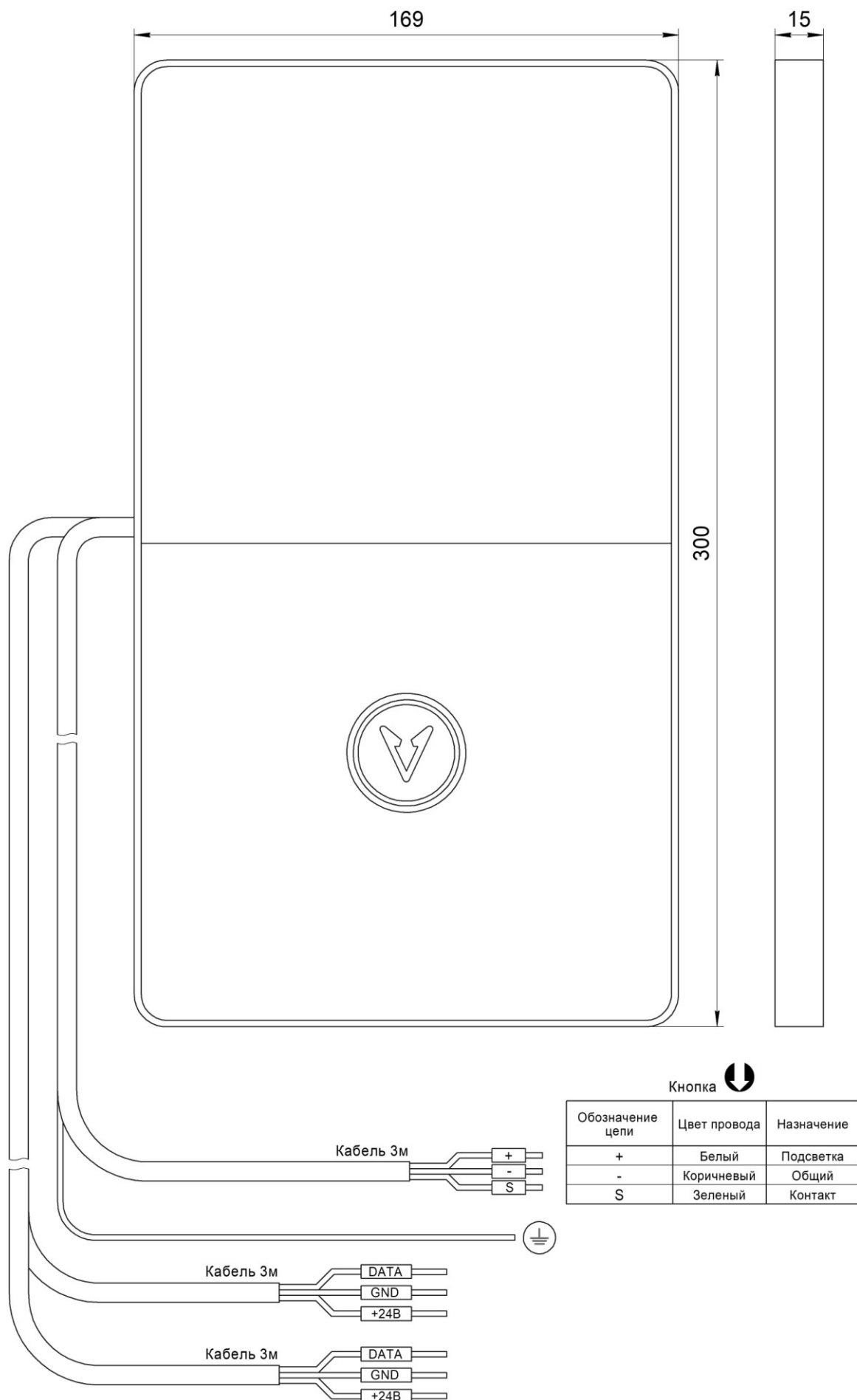
Рис.1 Внешний вид Вызывной пост ОНИКС НШЕК.468381.065-01
